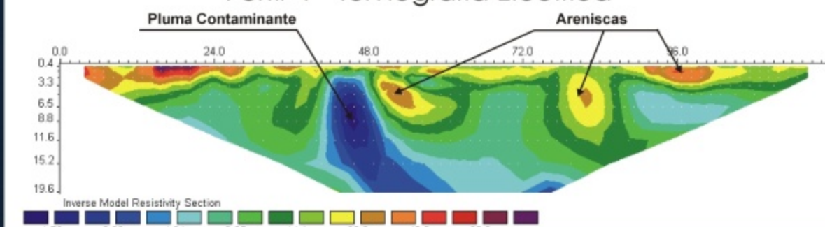
Perfil 4 - Tomografía Eléctrica
