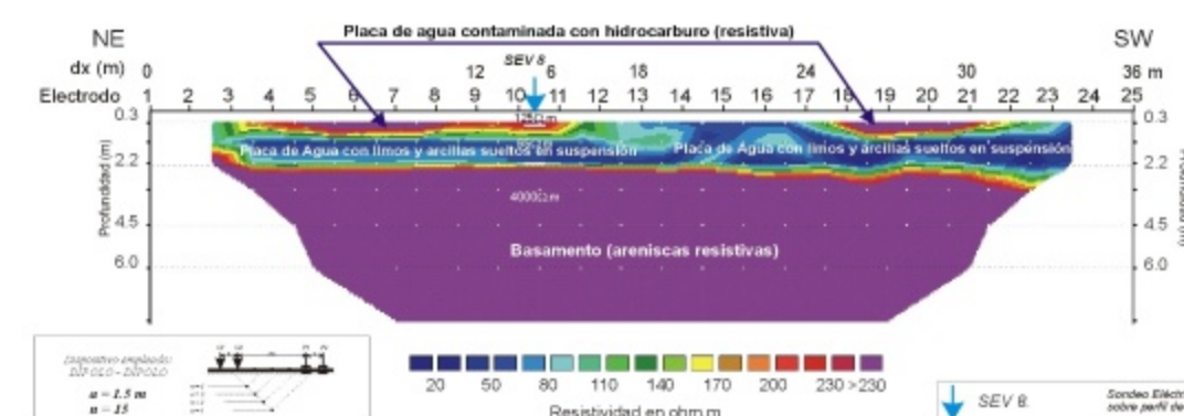
Tomografía Eléctrica Perfil N° 4 Sobre Placa de Agua
